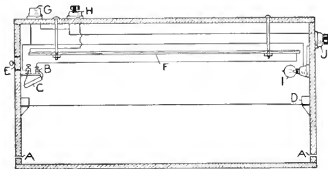
Fig. 1—Box Details
